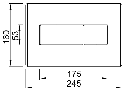
STY-800-1 fehér műanyag / white plastic / biele / alb / bijelo / белая
