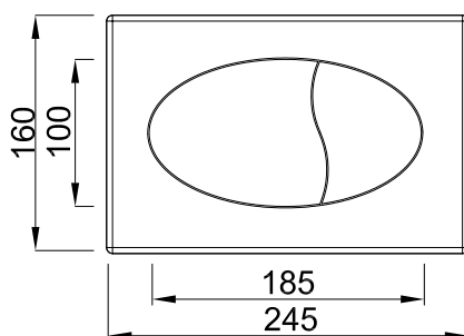
STY-801-1 fehér műanyag / white plastic / biele / alb / bijelo / белая
