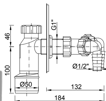
STY-511 rozsdamentes acél / stainless steel / krytom / inox / inox / нержавеющей стали
