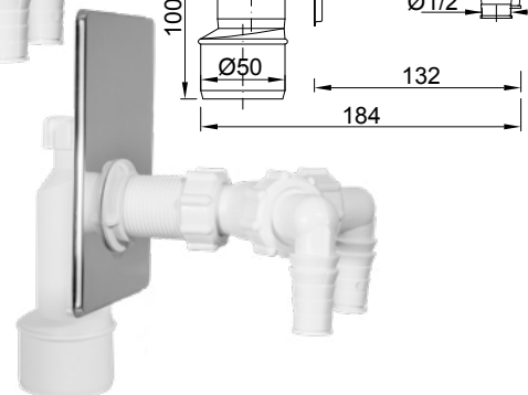
STY-511-Y rozsdamentes acél / stainless steel / krytom / inox / inox / нержавеющей стали
