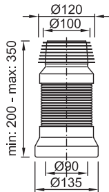
STY-530-F-R Rövid flexibilis WC bekötő Short adjustable length WC connector
