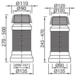
STY-530-F STY-530-F-Blue Flexibilis WC bekötők Adjustable length WC connector
